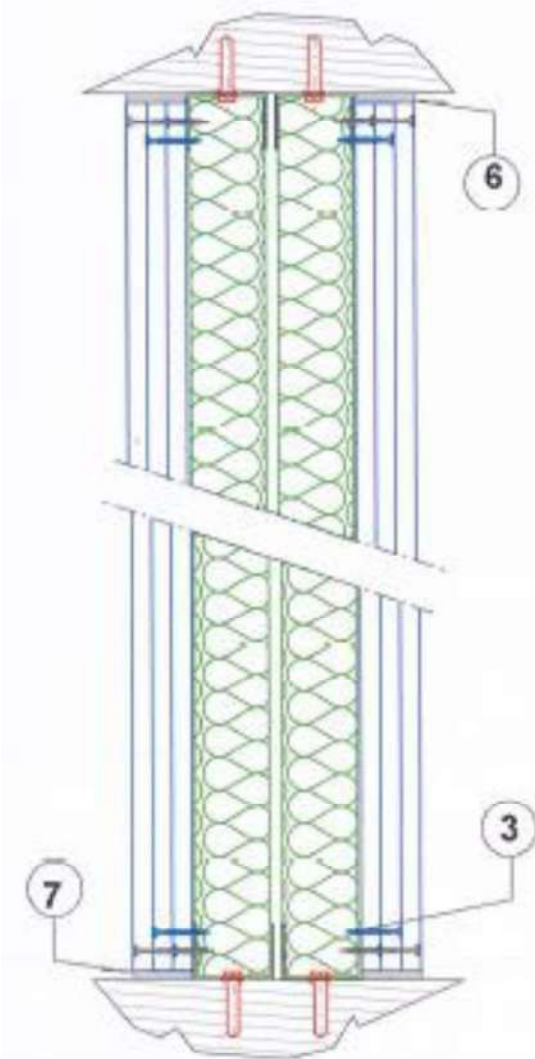
Coupe Verticale Cloison SAD 180 en BA 13
