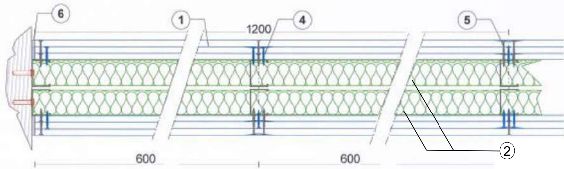
Coupe Horizontale Cloison SAD 180 en BA 13
